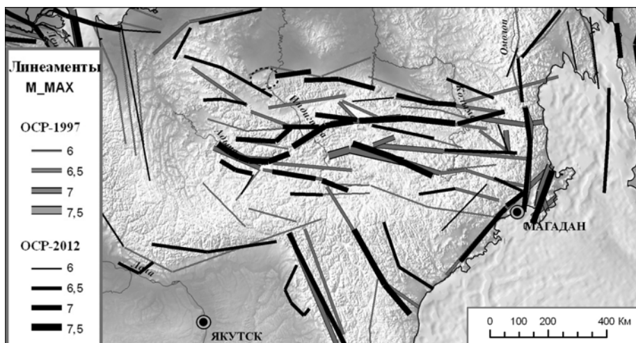
Рис. 3. Сейсмолинейменты разных M_{max} в моделях зон ВОЗ при создании карт ОСР-97 и ОСР-2012.
