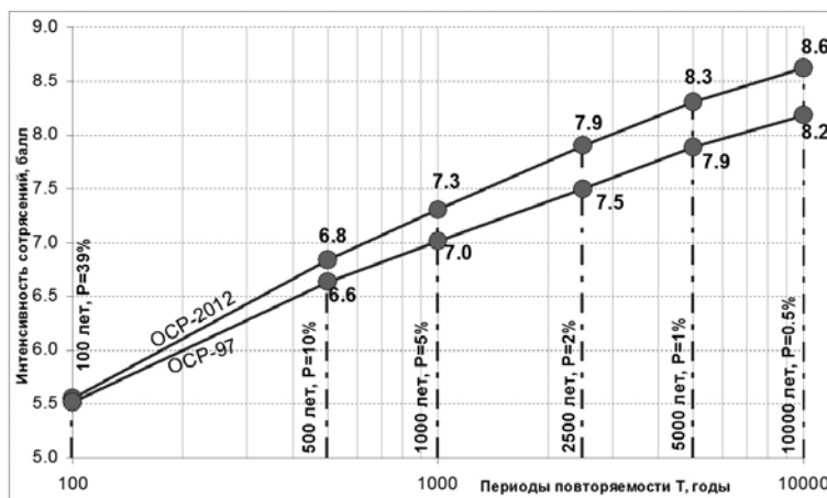
Рис. 2. Графики динамики сейсмической опасности для района эпицентра землетрясения 14.02.2013 г.
