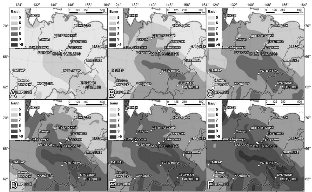
Рис. 1. Фрагменты карт ОСР-2012 (А, В, С, D, Е, F) для территории Республики Саха-Якутия, запада Магаданской области и севера Хабаровского края (показаны административные границы между ними).
