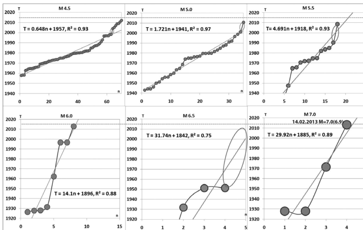
Рис. 5. Графики накопления сейсмических событий разных магнитуд на территории региона 4.4.
