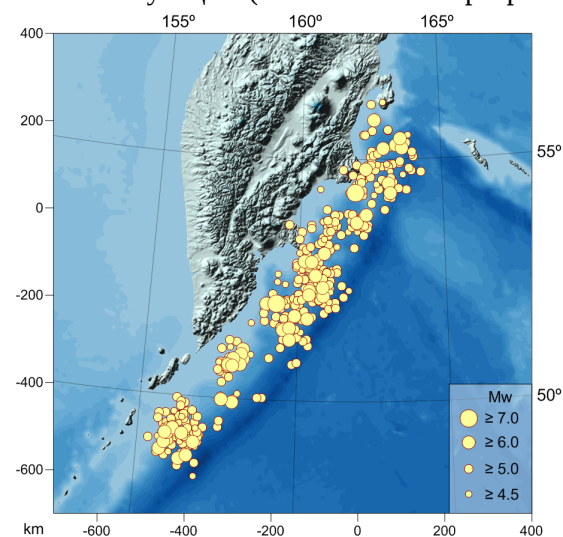
Рис. 1. Эпицентры центроидов субдукционных землетрясений, использованных для построения эмпирических вероятностных распределений параметров механизмов землетрясений.
