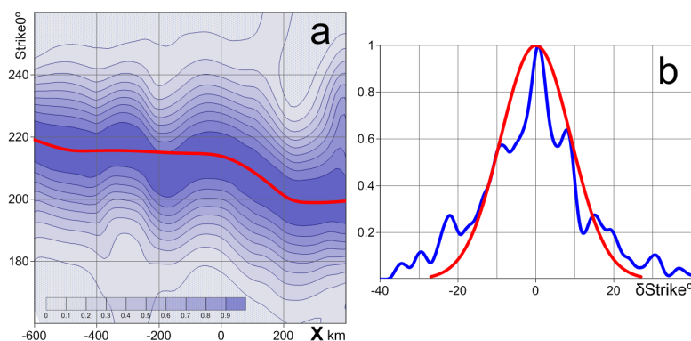
Рис.4. Построение распределения для генерирования простираия разрыва в механизме модельного очага. Обозначения аналогичны рис.3. В гистограмме а каждое сечение, параллельное оси Strike нормировано на частный максимум. Пояснения в тексте.
