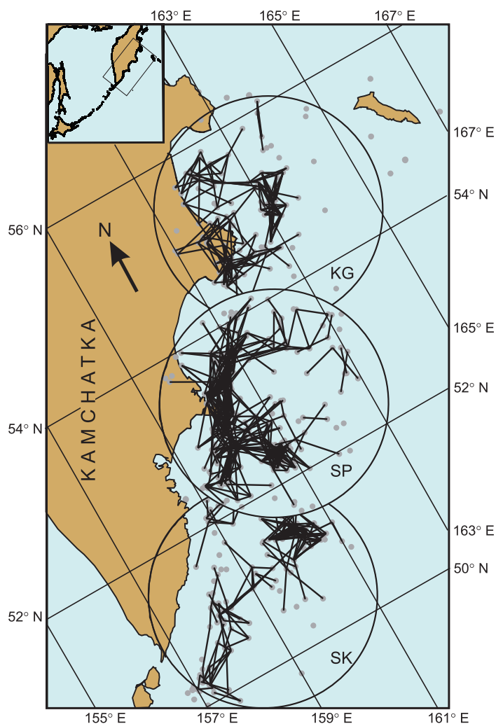
Рис. 1. Примеры расположения пар эпицентров для трех изученных кругов – SP, SK и KG (1962 г.). Параметры выделения пар следующие: (\Delta t_1 \Delta t_2)=0-15 сут, (D_1 D_2)=15-60 км, K^{\Phi 68}=8.5-11.4 ( M_L=3.5-5.0 ). Расположение района работ – на врезке.
